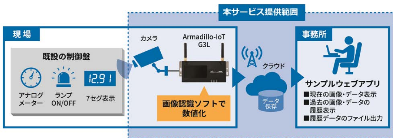
「メーター読み取り」のシステム構成図
